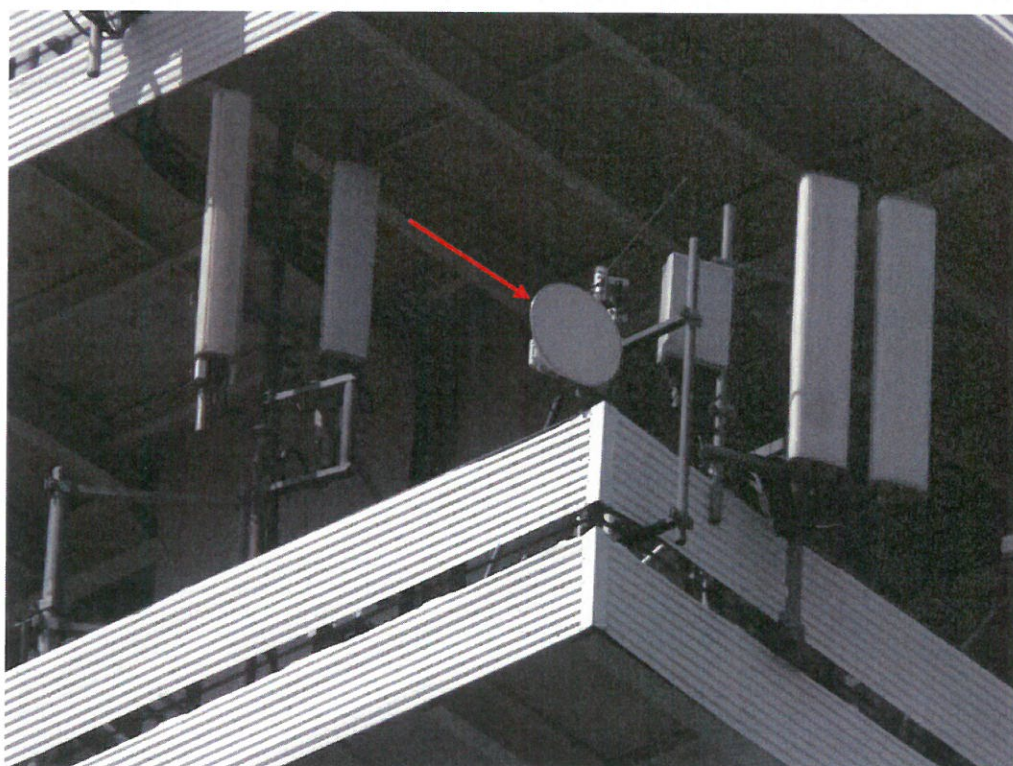
Widok instalacji radiokomunikacyjnej Stacja Netia RZEB031 - RZEM00010 Rzeszów, ul. Władysława Broniewskiego 1.
